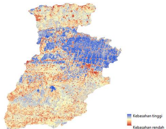
Gambar 2. Hasil pengolahan metode NDWI Kabupaten Lamongan
