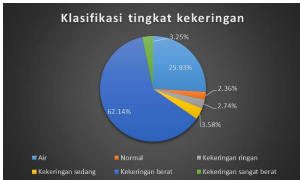
Gambar 7. Presentase hasil pengolahan NDDI Kabupaten Lamongan
